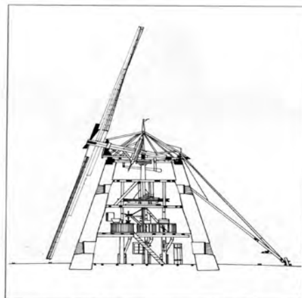
208. A Sáfrók Malom metszete. Nagy Szeder István rajza. Mendele Ferenc - Németh B. Ferenc 1967. 218. alapján
